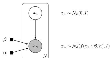
Fig. 1: Non-linear PCA
